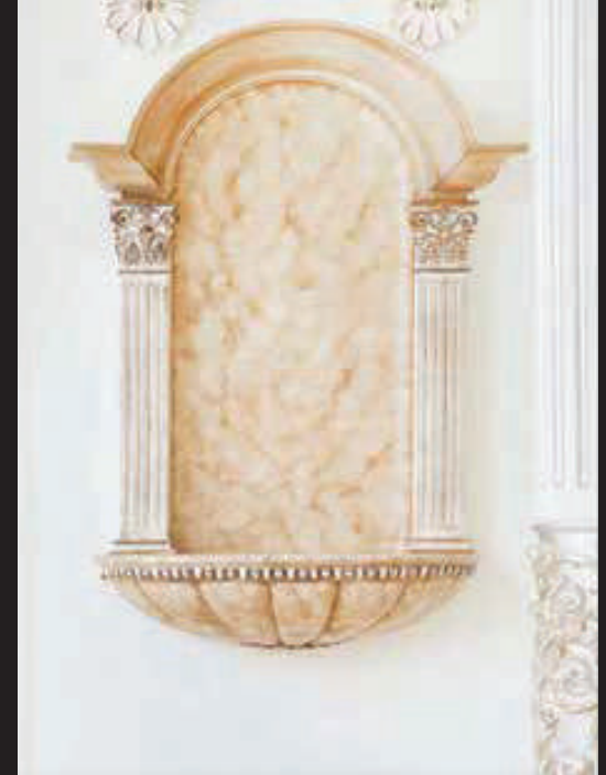
▲ PU-NİŞ-001 A: 592 mm B: 532 mm C: 385 mm D: 822 mm E: 108 mm F: 146 mm G: 202 mm H: 132 mm
